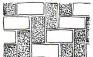
Elleboogverband Eigenlijk een Keperverband maar dan niet diagonaal gelegd.
